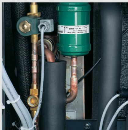
Rys. 18: Przeważacz gazu zasysanego w pompie ciepła Vitocal 300
