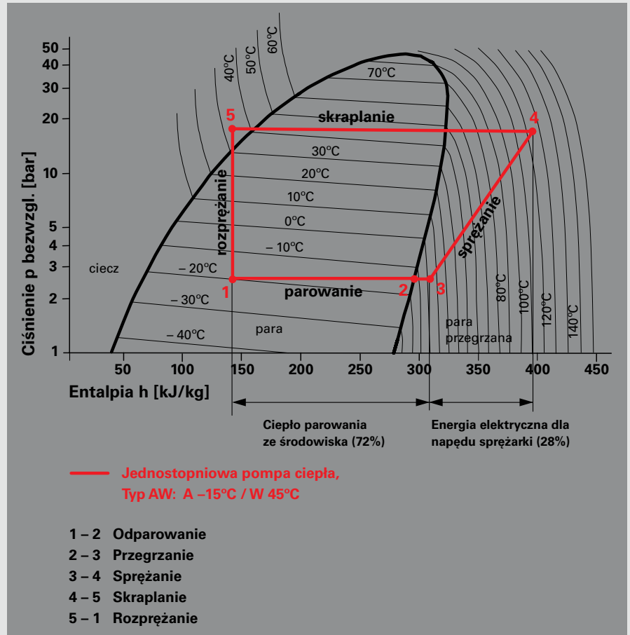
Rys. 17: Wykres lg p-h dla przeważacza
