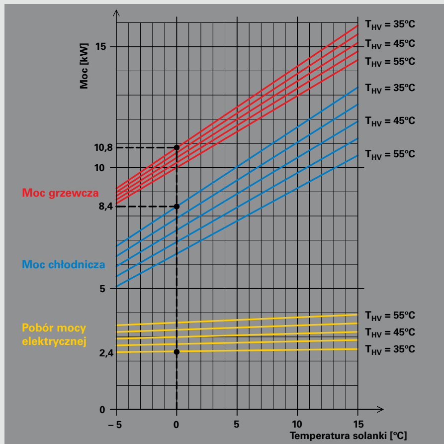
Rys. 11: Wykres mocy Vitocal 300, typ BW 110
