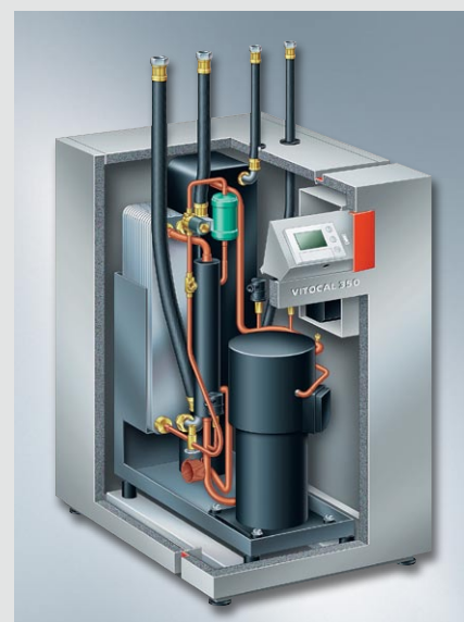
Rys. 52: Vitocal 350 z temperaturą zasilania 65°C
