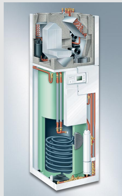
Rys. 34: Vitotres 343 – kompaktowa centrala grzewcza dla domów pasywnych, kombinowana z mechaniczną wentylacją pomieszczeń i pojemnościowym podgrzewaczem c.w.u.
