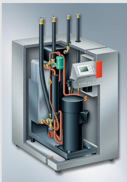
Rys. 8: Pompa ciepła solanka/woda Vitocal 300
