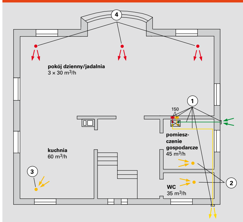
Rys. 13. Przykładowe rozmieszczenie zaworów powietrza doprowadzanego i użytego
