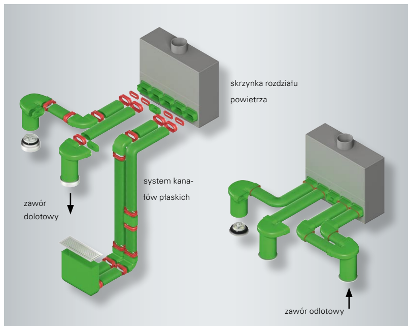
System płaskich kanałów z tworzywa sztucznego do szybkiego i łatwego montażu
