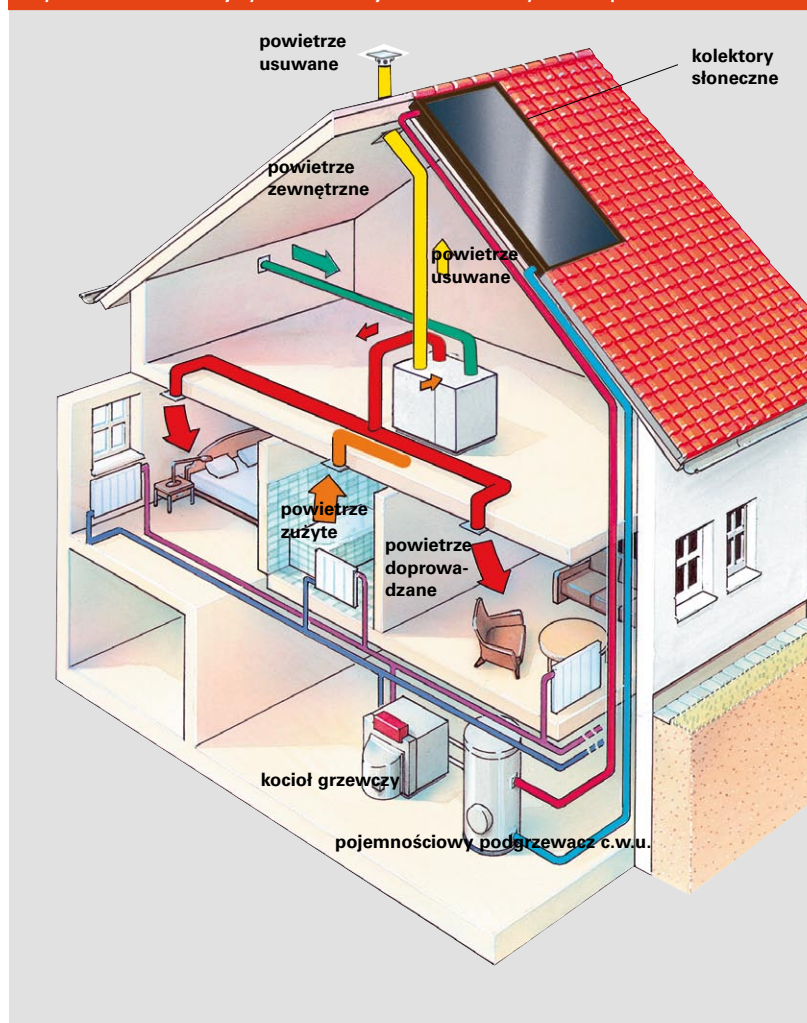
Rys. 1. Schemat instalacji systemu wentylacji mieszkania z odzyskiem ciepła
